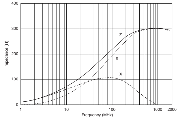
BLM18EG221TH1
